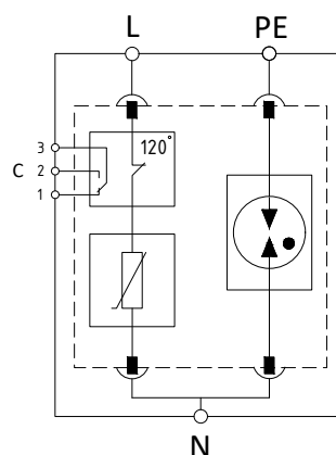
Принципиальная схема
