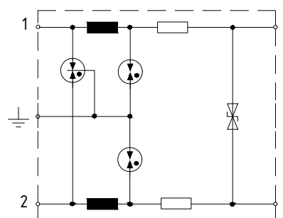
Принципиальная схема
