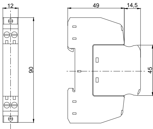
Габаритные размеры
