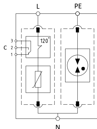
Принципиальная схема
