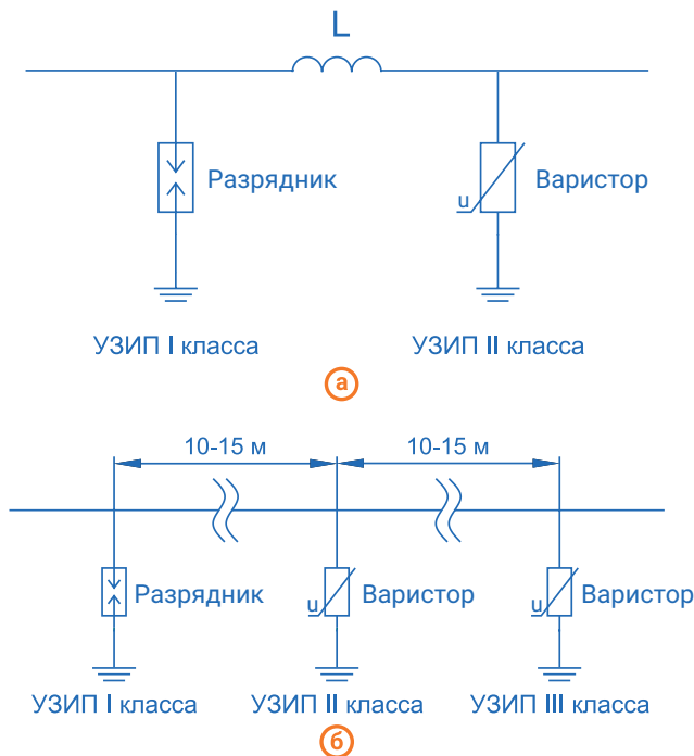
Рис. 10. Обеспечение селективной работы УЗИП: а) катушка индуктивности в качестве развязывающего элемента; б) провод в качестве развязывающего элемента.
