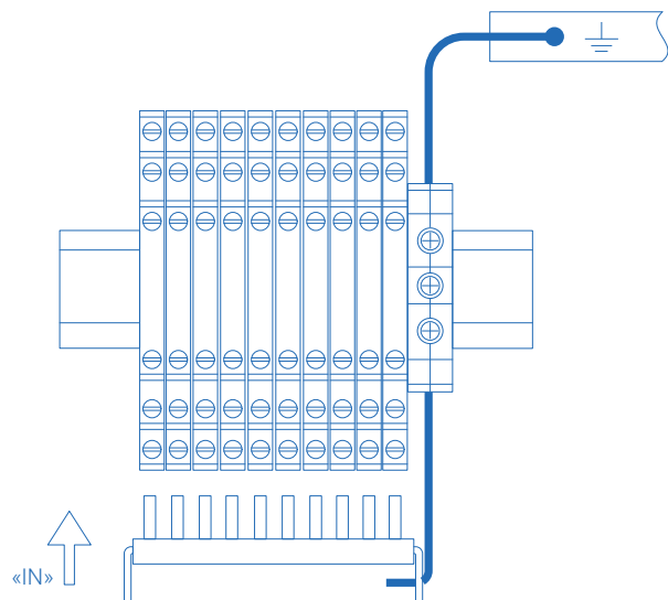
Рис. 30. Заземление группы УЗИП с помощью медного шинпровода
