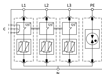
Принципиальная схема
