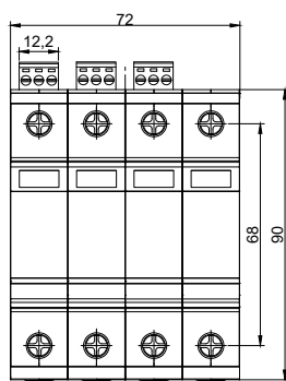
Габаритные размеры
