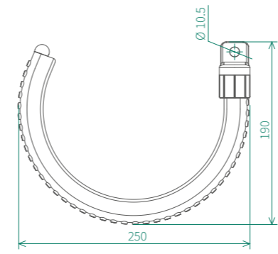
Габаритные размеры РМК-20
