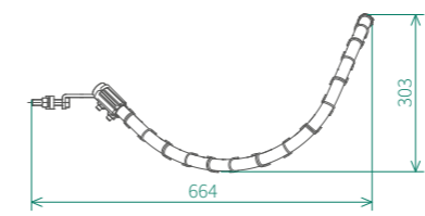
Габаритные размеры РДИП-10
