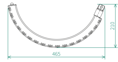
Габаритные размеры РМКЭ-10
