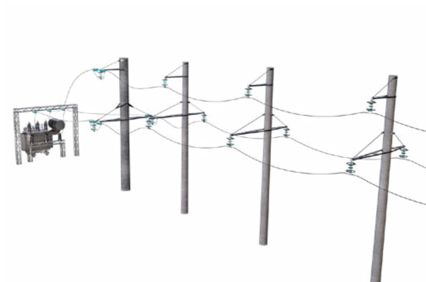
Рис. 29. Защита подхода ВЛ 35 кВ к подстанциям
