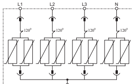
Принципиальная схема
