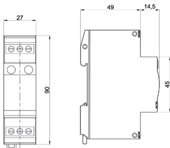
Габаритные размеры
