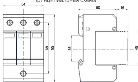
Габаритные размеры
