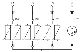
Принципиальная схема
