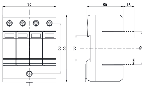
Габаритные размеры
