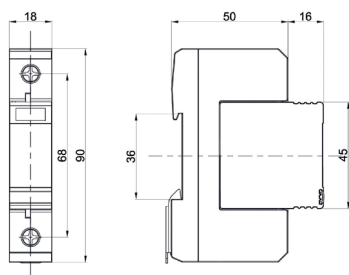
Габаритные размеры
