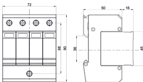
Габаритные размеры
