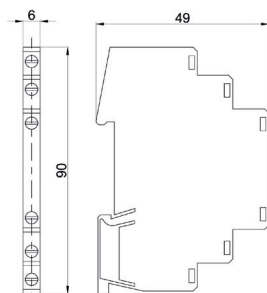
Габаритные размеры
