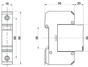
Габаритные размеры
