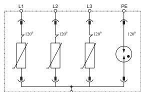
Принципиальная схема
