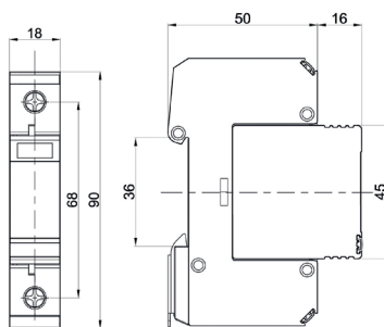
Габаритные размеры
