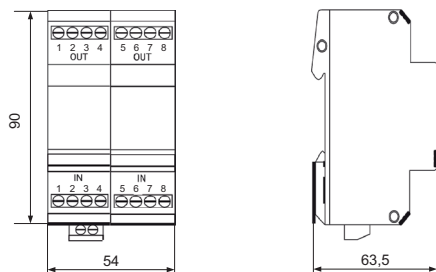
Габаритные размеры
