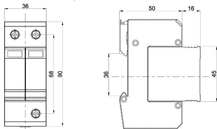
Габаритные размеры
