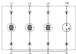
Принципиальная схема
