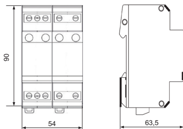
Габаритные размеры
