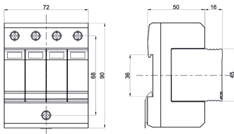
Габаритные размеры
