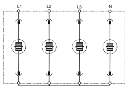
Принципиальная схема
