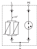
Принципиальная схема
