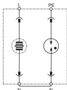
Принципиальная схема
