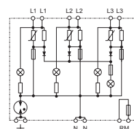
Принципиальная схема
