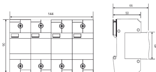
Габаритные размеры
