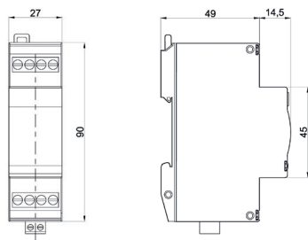
Габаритные размеры
