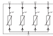
Принципиальная схема
