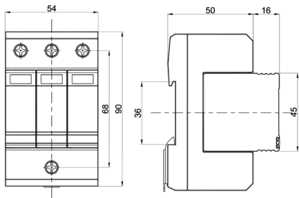
Габаритные размеры
