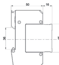
Габаритные размеры
