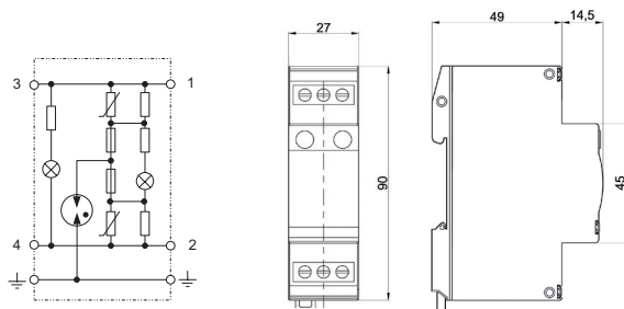
Принципиальная схема
