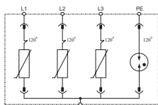
Принципиальная схема
