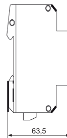
Габаритные размеры
