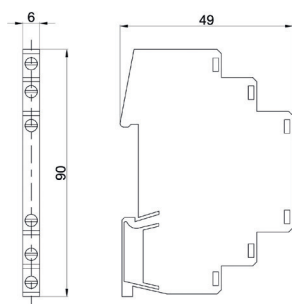
Габаритные размеры
