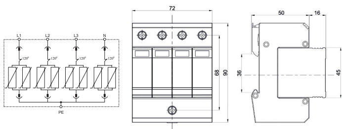
Принципиальная схема
