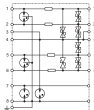
Принципиальная схема
