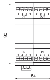
Габаритные размеры
