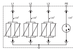
Принципиальная схема
