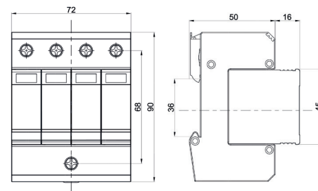
Габаритные размеры
