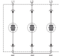
Принципиальная схема
