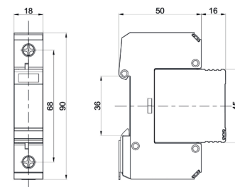
Габаритные размеры
