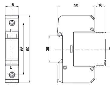
Габаритные размеры
