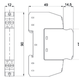
Габаритные размеры
