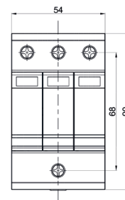
Габаритные размеры
