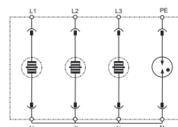
Принципиальная схема
