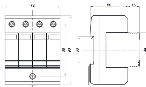
Габаритные размеры
