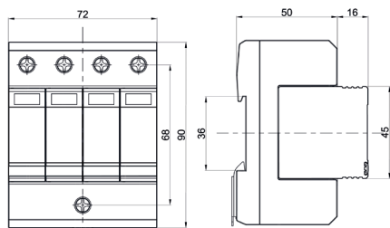
Габаритные размеры
