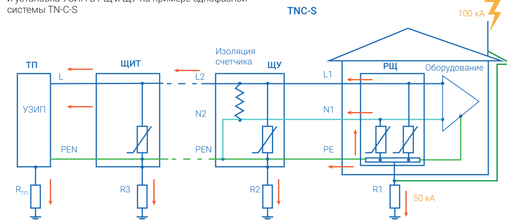
Рисунок 2 - ПУМ в объект. Растекание тока молнии и установка УЗИП в РЩ и ЩУ на примере однофазной системы TT
